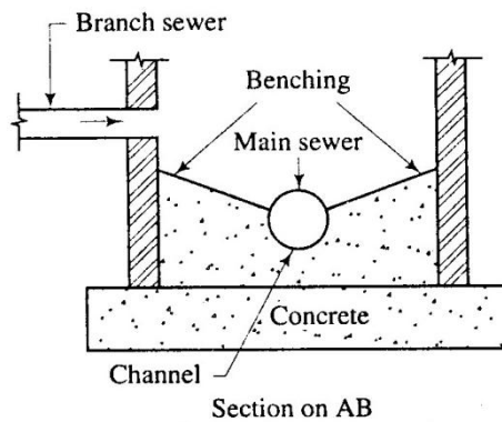
Bottom of manhole
