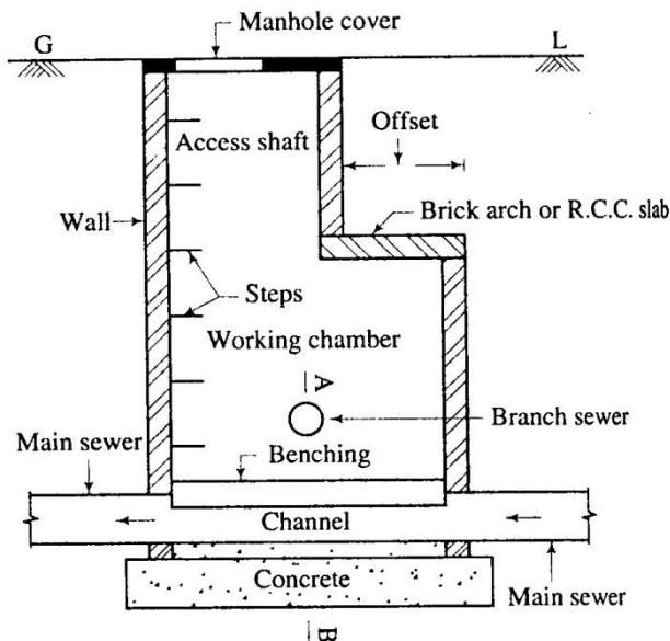
Deep manhole
